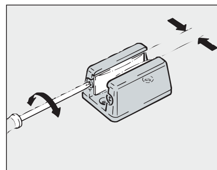
Guidage au sol sans jeu. Réglage de 8 - 12,7 mm.
