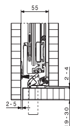
Connector: 55 mm épaisseur maximum par porte: 19-30 mm
