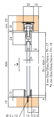
sans rail inférieur GPK
