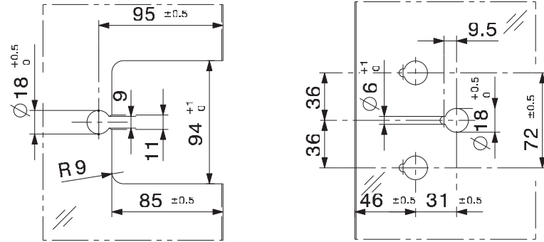
avec partie fixe
