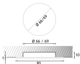
Dessin technique (bois)
