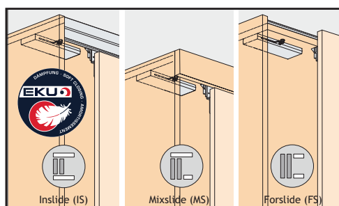
Amortissement avec retrait en option
