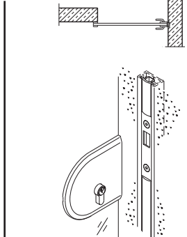
avec profil mural
