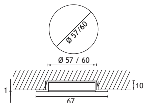
Dessin technique
