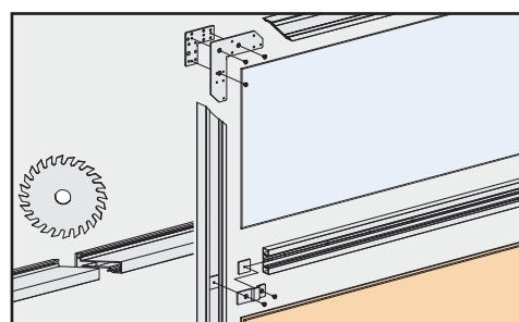
Simplicité de confection du cadre
