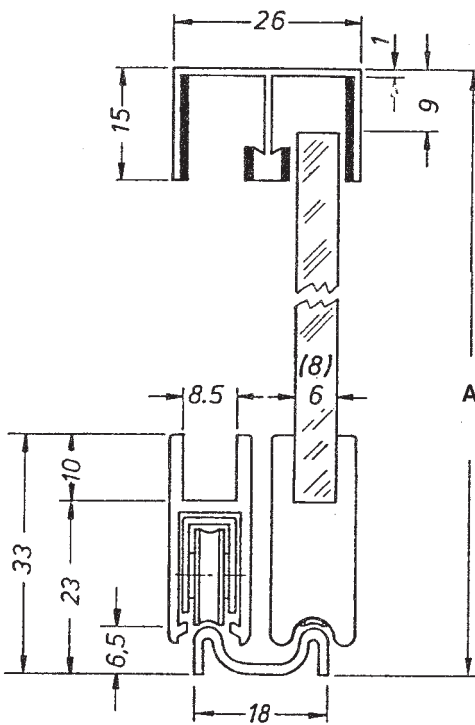
Hauteur de la porte= A-32 mm
