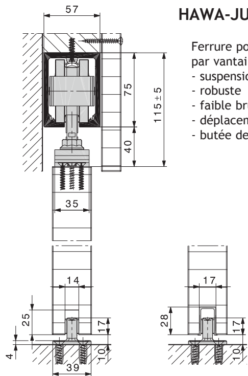
sans profil de guidage avec profil de guidage
