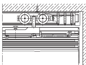
montage avec clavette de montage
