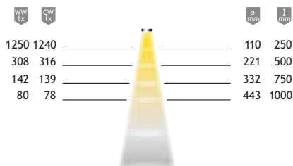
Diagramme de répartition de lumière 25°
