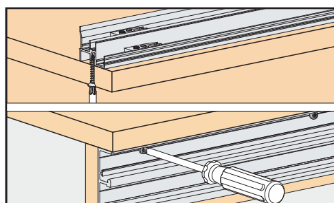
Montage ultérieur simple des rails
