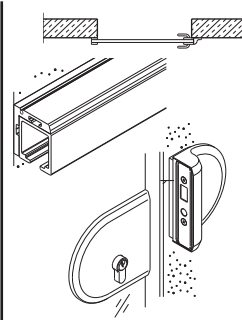
avec fixation murale
