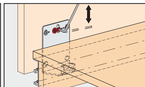
Ajustement en hauteur confortable
