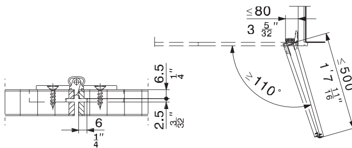
fraisage du profil de liaison
