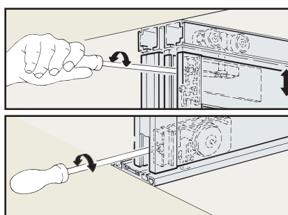
Réglage en hauteur intégré.
