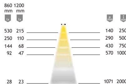
Diagramme de répartition de lumière 30°
