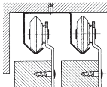
Epaisseur de porte: 28 à 33 mm
