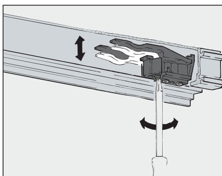
Réglage en continu de la force de blocage.
