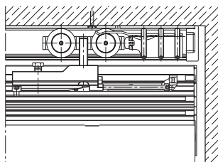
montage avec clavette de montage
