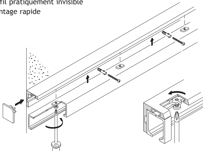
Profil en équerre pour montage mural simple du Junior 40, 80 et 120/GP
