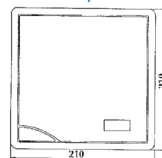
profondeur d'encastrement: 30 mm Découpe lxp: 195 x 195 mm
