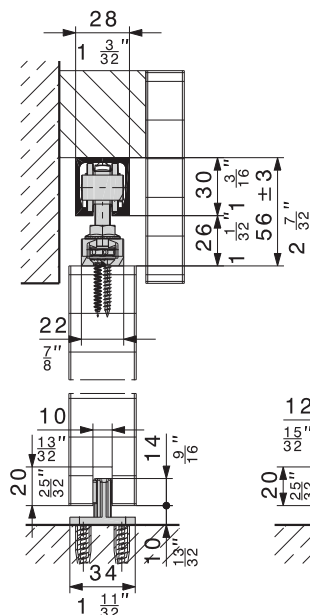
sans profil de guidage avec profil de guidage
