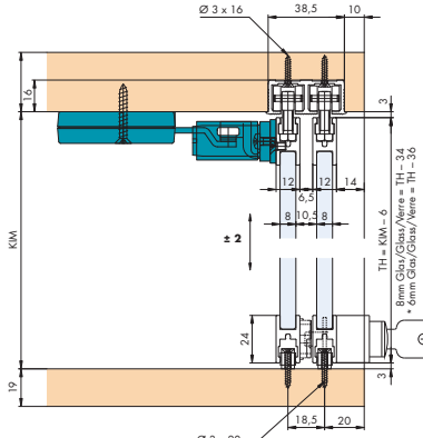
avec rail inférieur GPPK
