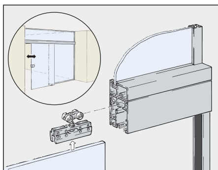
Système de vitrage pour le montage entre parois avec imposte (Porta GWF/GW/GFO).
