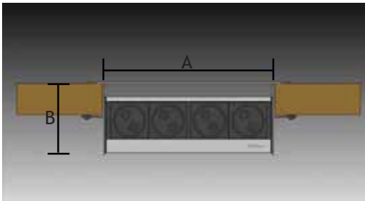
Dimensions d'encastrement: A= L:227 mm x l:157 mm B= max. 95 mm
