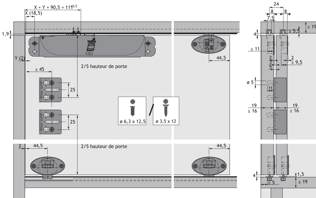
SlideLine 55 Plus avec Silent System / porte rentrante
