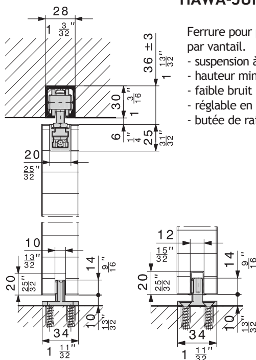
sans profil de guidage avec profil de guidage
