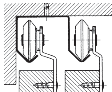
Epaisseur de porte: 23 à 28 mm
