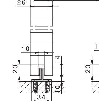
sans profil de guidage
