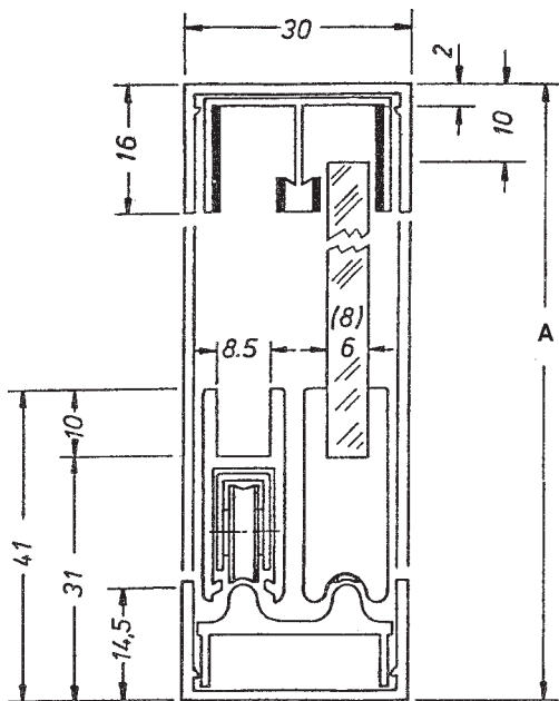
Hauteur de la porte= A-41mm
