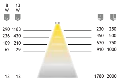
Diagramme de répartition de lumière 48°
