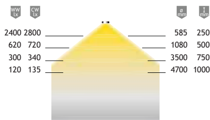
Diagramme de répartition de lumière 120°
