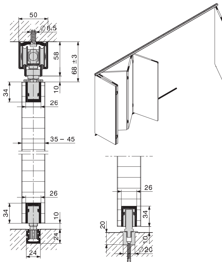
Ferrure pour grandes parois pliantes en bois, jusqu'à un poids de porte de 80 kg.
