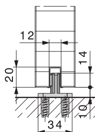
avec profil de guidage
