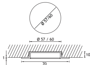
dessin technique
