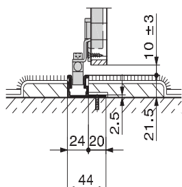
fraisage du profil de liaison
