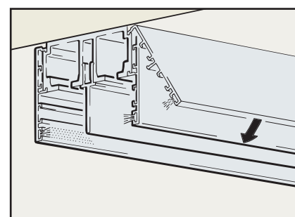
Cache design à clipser pour rail de roulements.
