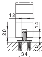
avec profil de guidage
