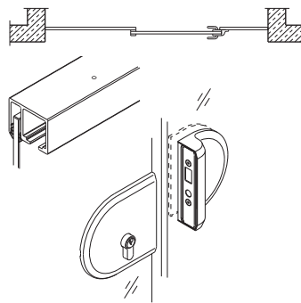
avec partie fixe
