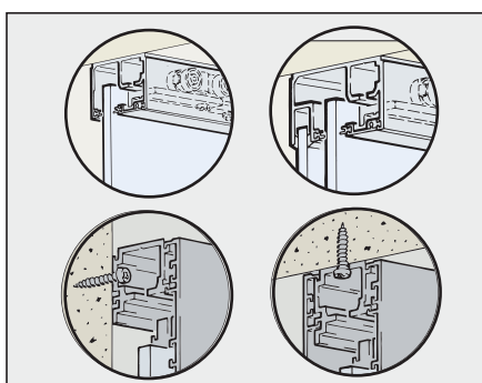
Rail de roulement pour montage mural ou au plafond.
